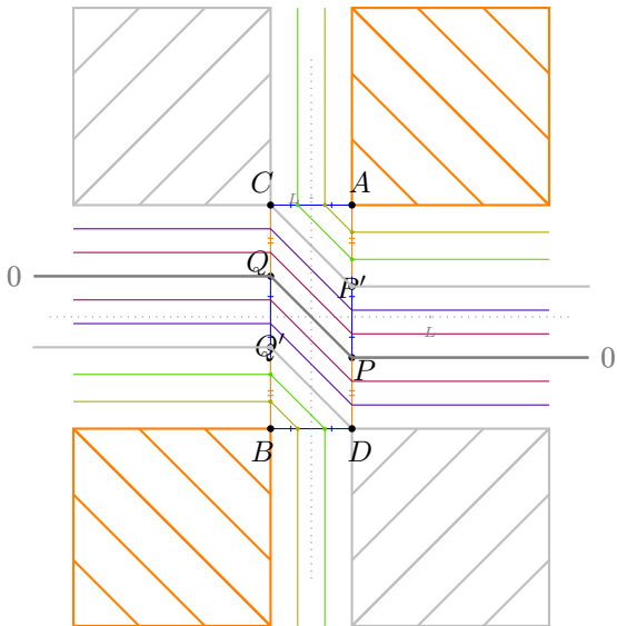
Case: 2 \theta = 70.0
