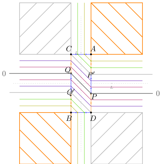
Case: 2 \theta = 71.0
