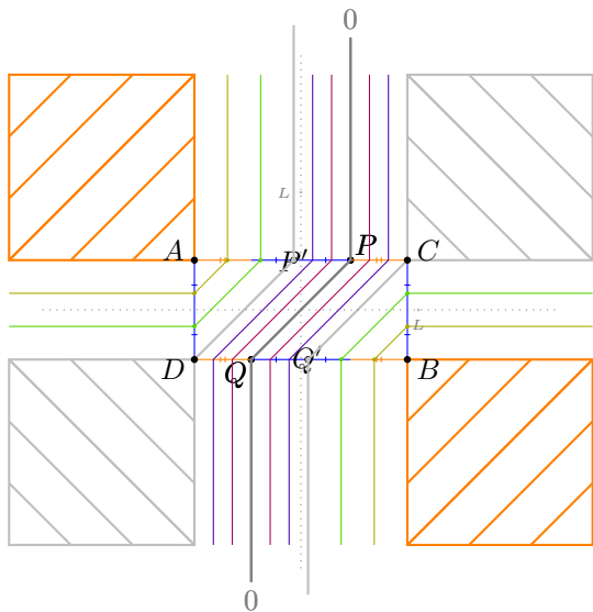
Case: 4 \theta = 155.0
